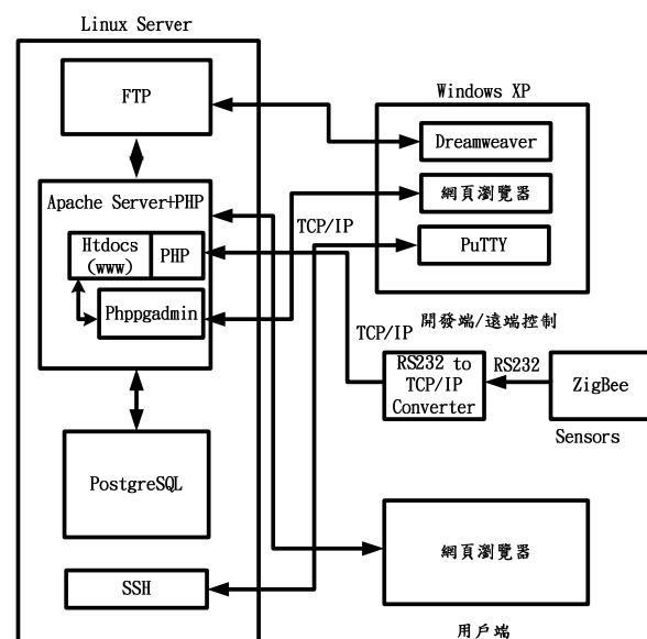
圖 8. 網頁式資料庫管理系統架構示意圖
