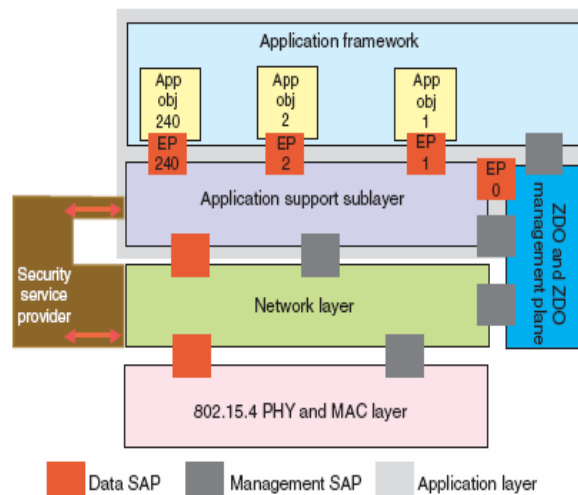
圖 6. 802.15.4 協議堆疊(stack)示意圖
