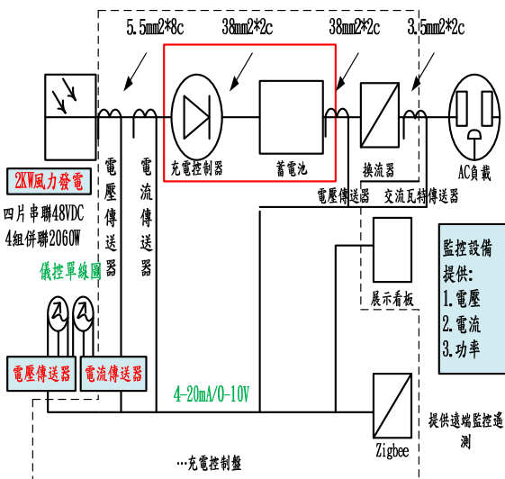
圖 3. 小型化垂直軸式風車風力發電系統感測器配置圖
