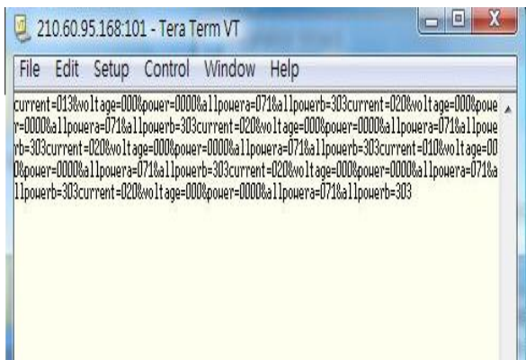
圖 11. 後端平台 ZigBee 接收量測之訊號值顯示
