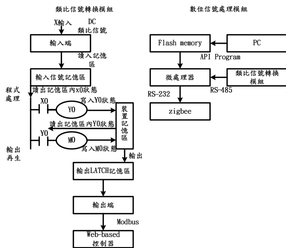
圖 5. 嵌入式資料擷取模組架構圖
