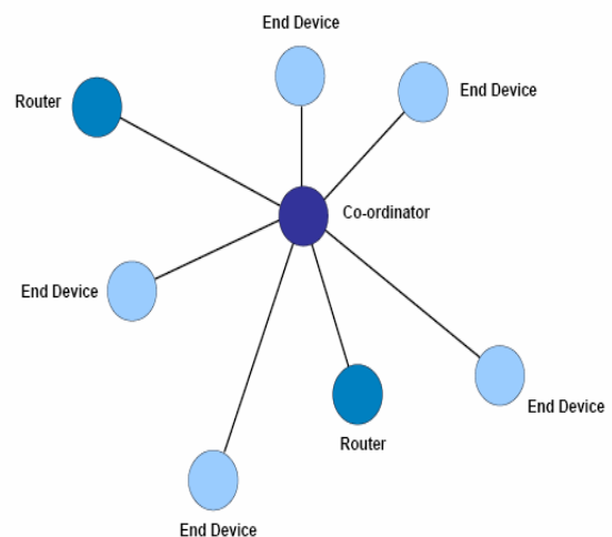
圖 7. Zigbee 星狀網路拓撲結構圖
