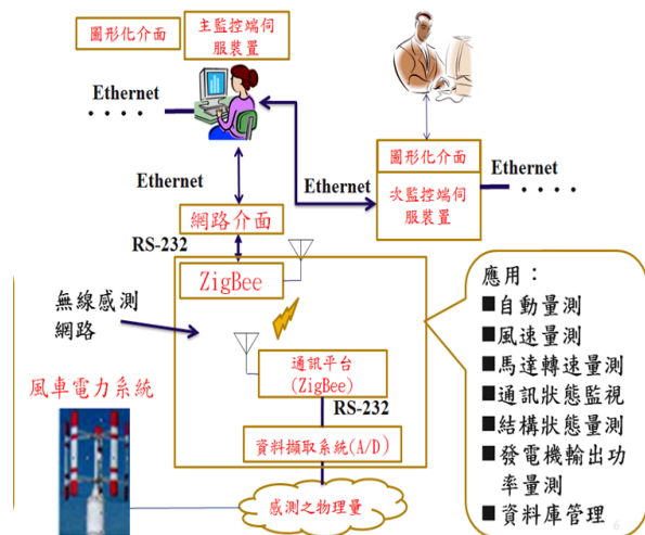
圖 2. 能源監控與網頁式資料庫管理系統
